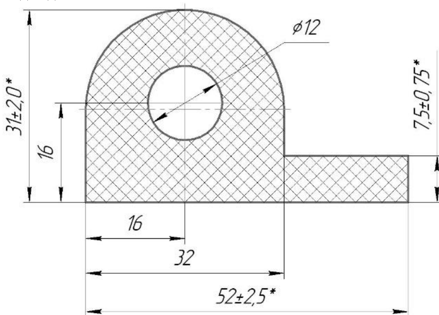
Рис. 1 – Резина уплотнительная (профильная) ТУСМ-8-01. Общий вид
