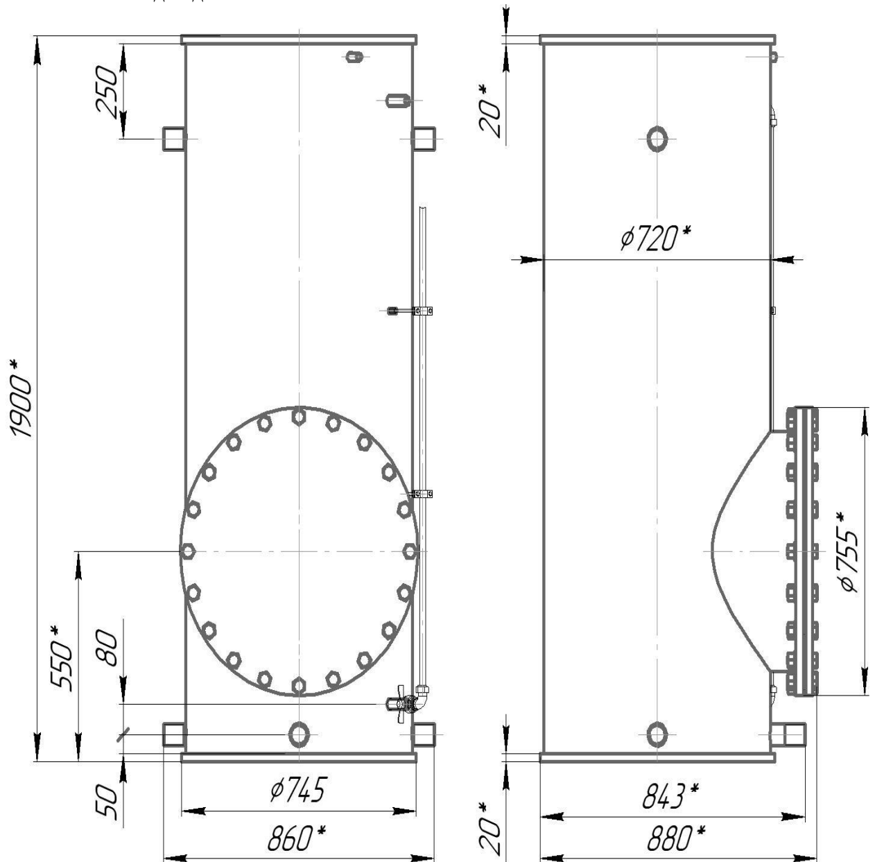
Рис. 1 - Бак для воды БВ-0,7БГ. Общий вид (с УУЖ – дополнительная комплектация).
