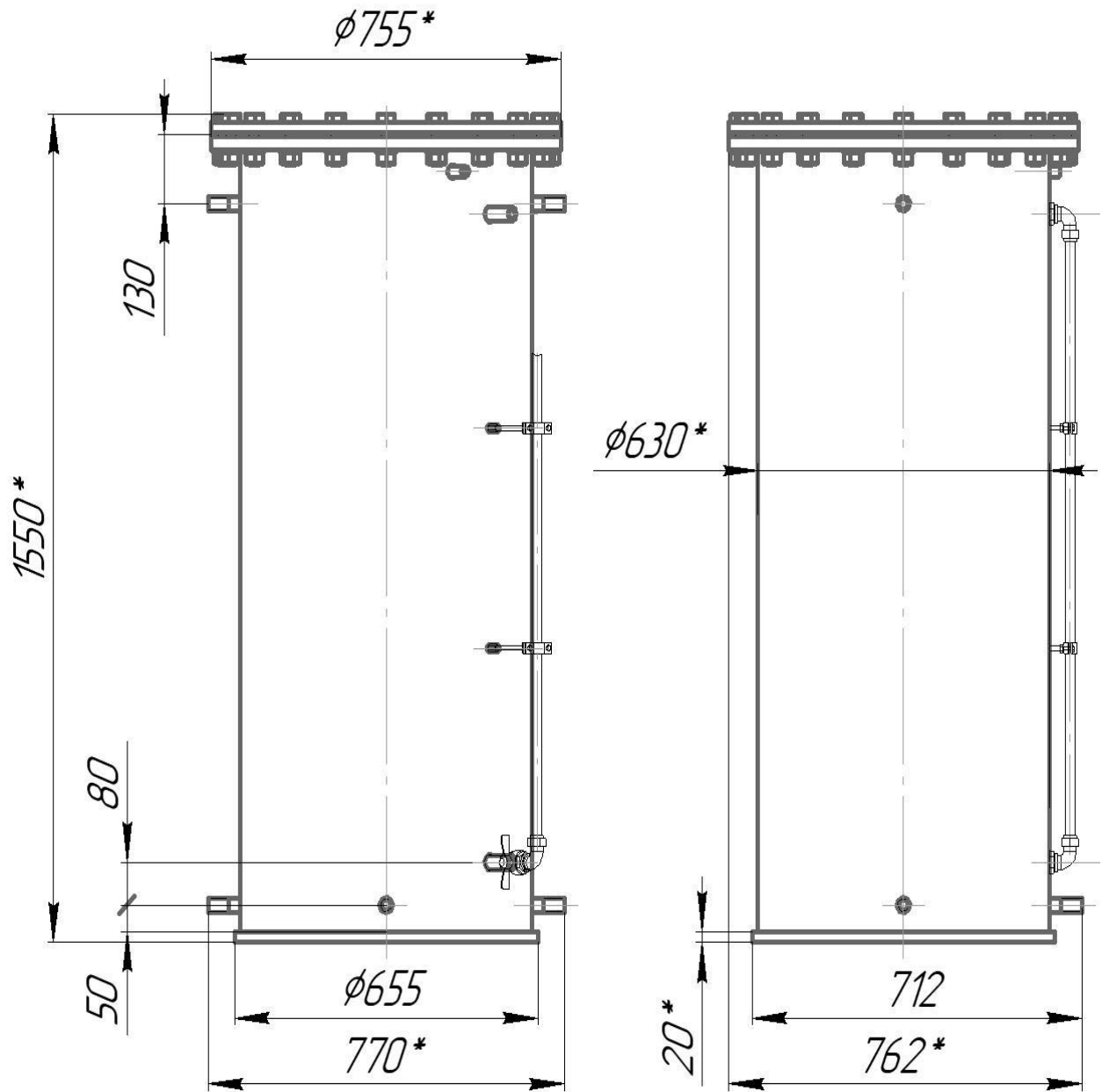
Рис. 1 - Бак для воды БВ-0,4. Общий вид (с УУЖ – дополнительная комплектация).
