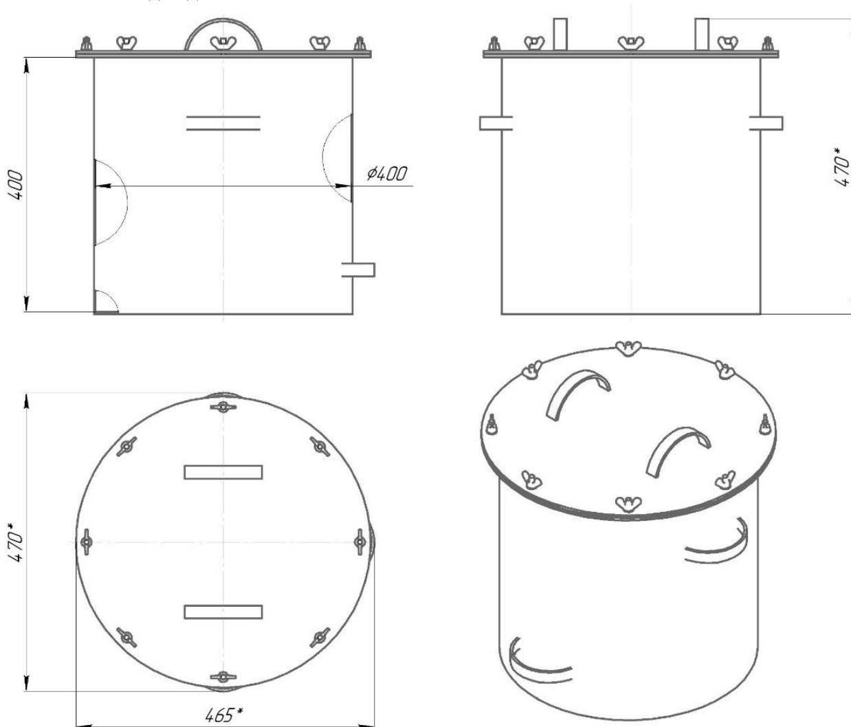
Рис. 1 - Бак инвентарный выносной БИВ-45. Общий вид.
