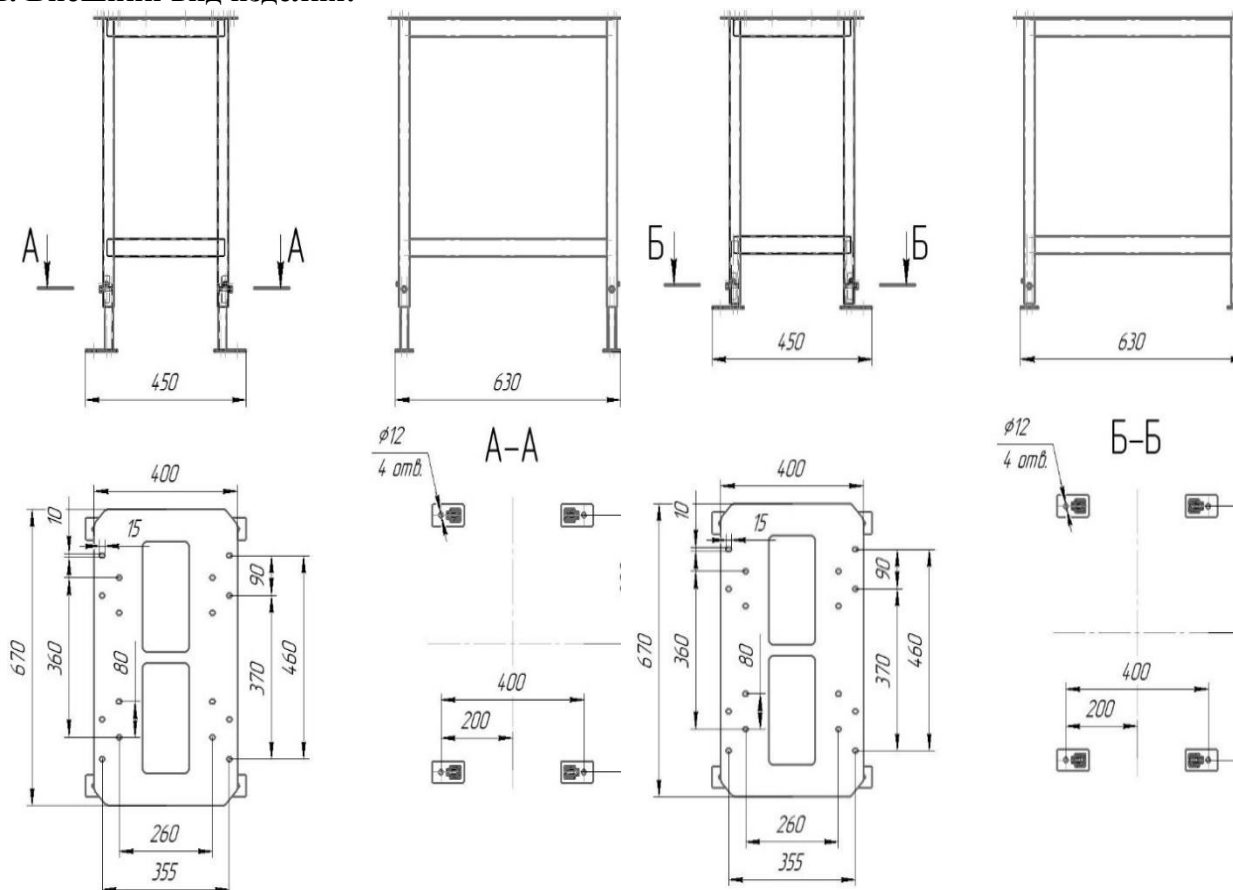
Рис. 1 – СВ-2 в положении для ЭРВ-72-2. Общий вид.
