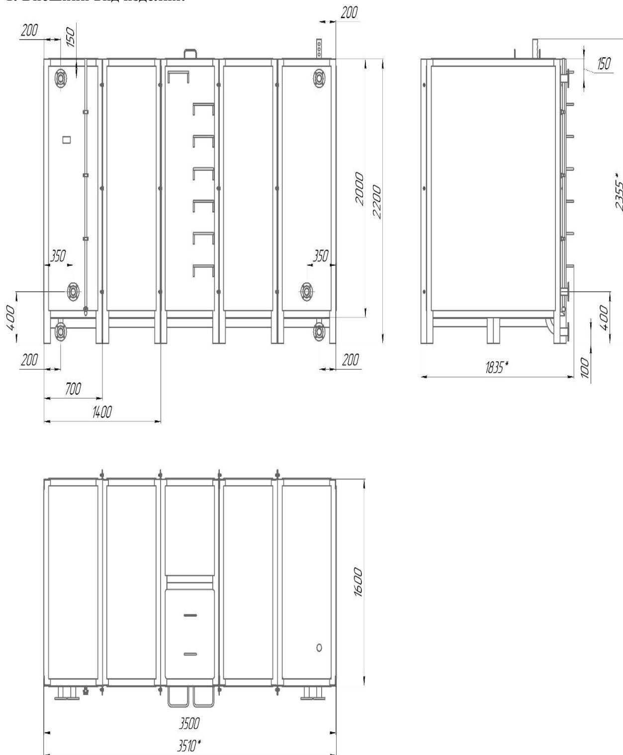
Рис. 1 - Бак для воды БВ-10. Общий вид (с УУЖ – дополнительная комплектация).
