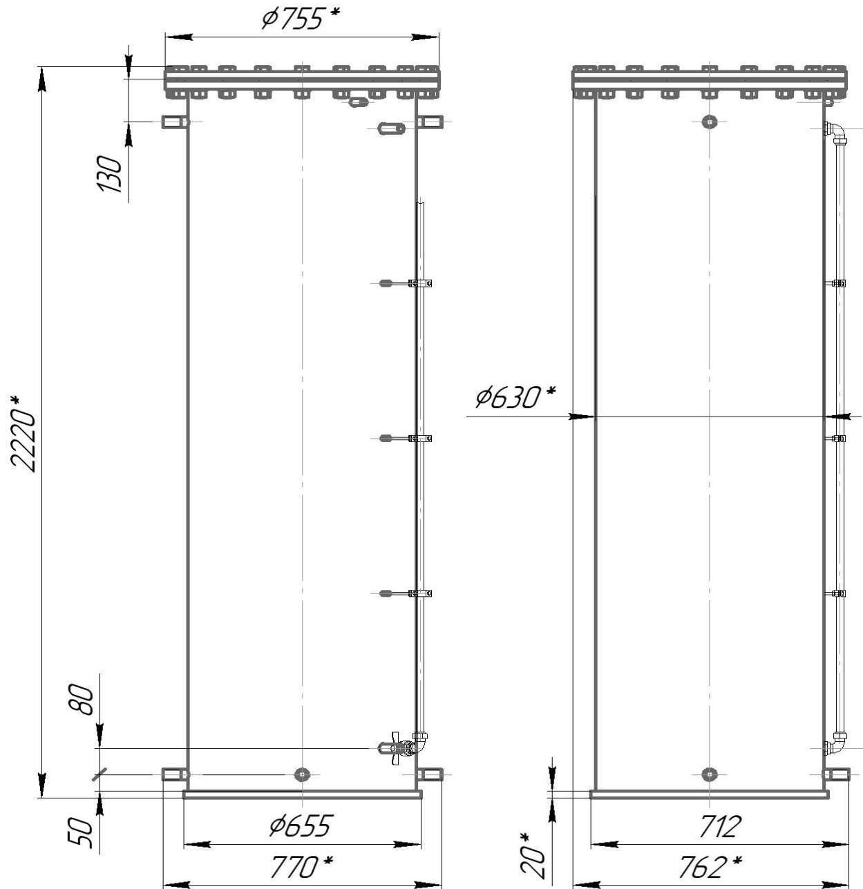
Рис. 1 - Бак для воды БВ-0,6. Общий вид (с УУЖ – дополнительная комплектация).
