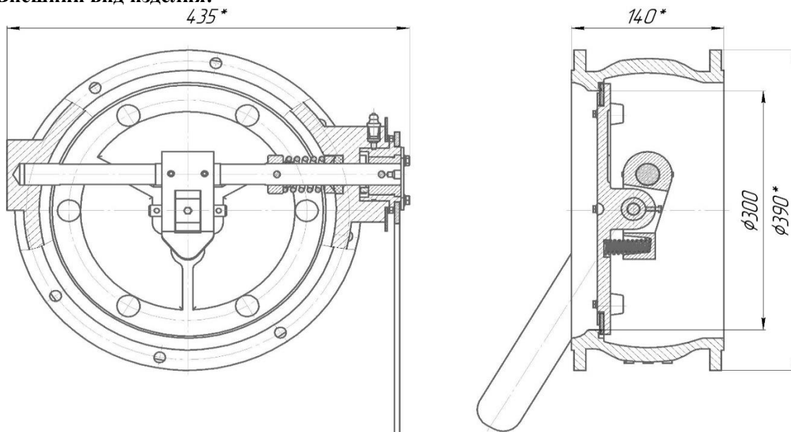
Рис. 1 - Клапан герметический КГ-300 в сборе. Общий вид
