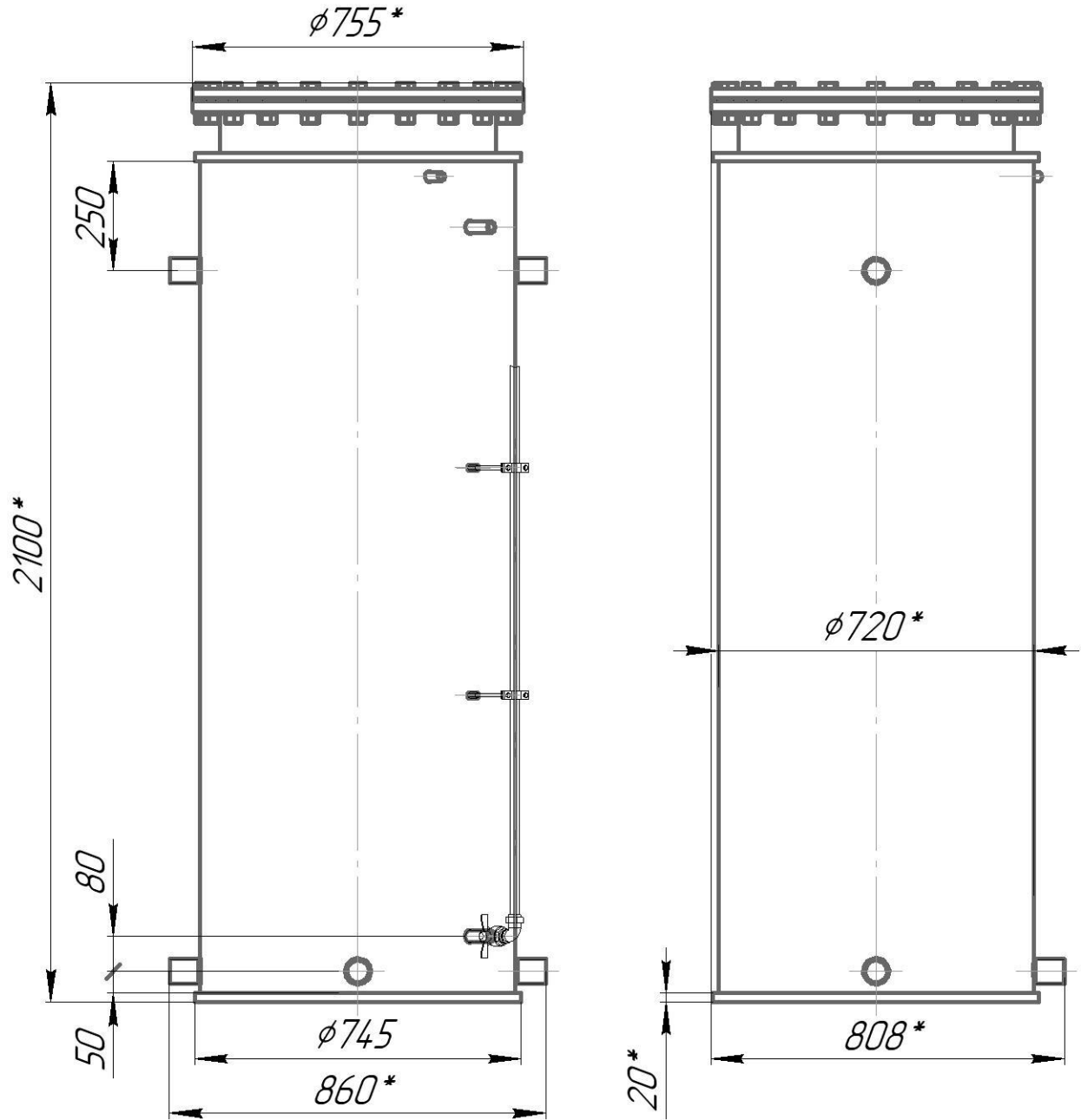
Рис. 1 - Бак для воды БВ-0,7. Общий вид (с УУЖ – дополнительная комплектация).
