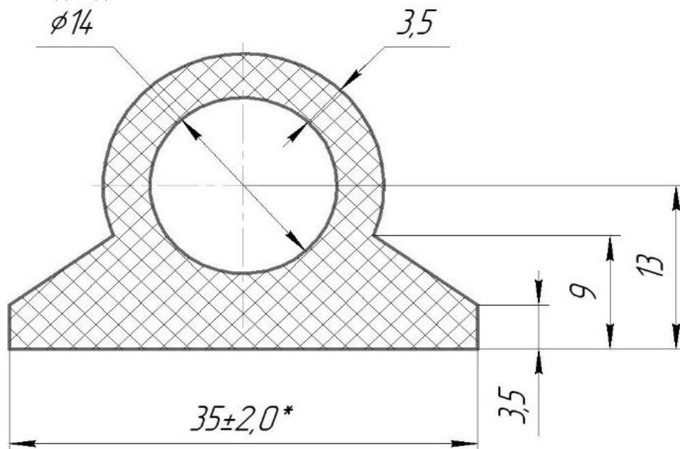
Рис. 1 – Резина уплотнительная (профильная) 86.029.03. Общий вид
