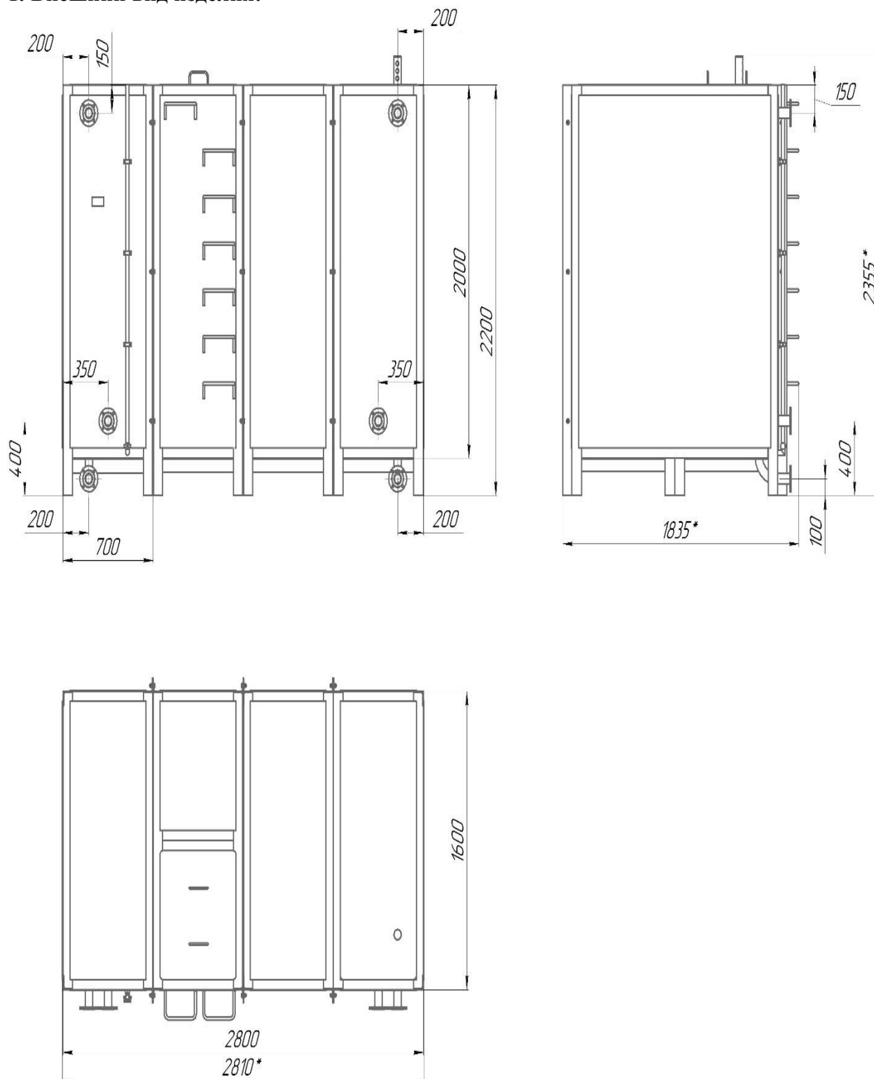
Рис. 1 - Бак для воды БВ-8. Общий вид (с УУЖ – дополнительная комплектация).
