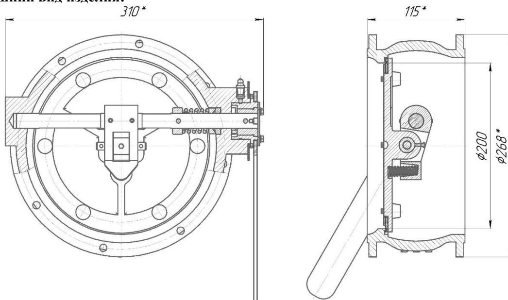
Рис. 1 - Клапан герметический КГ-200 в сборе. Общий вид
