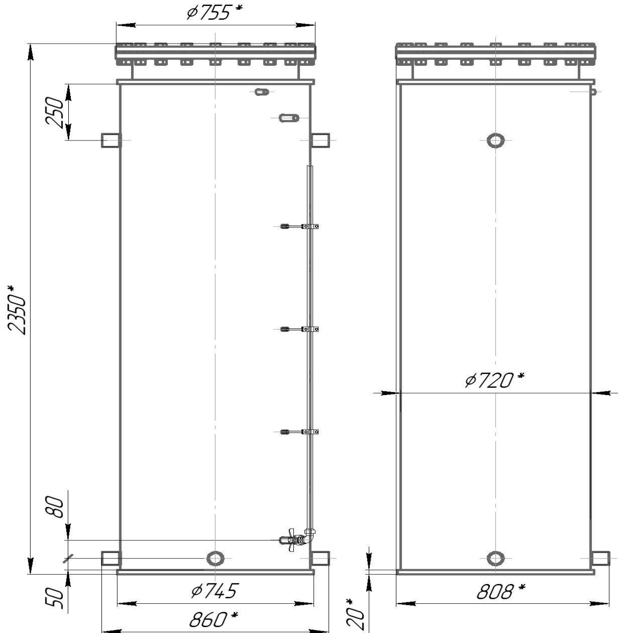
Рис. 1 - Бак для воды БВ-0,8. Общий вид (с УУЖ – дополнительная комплектация).
