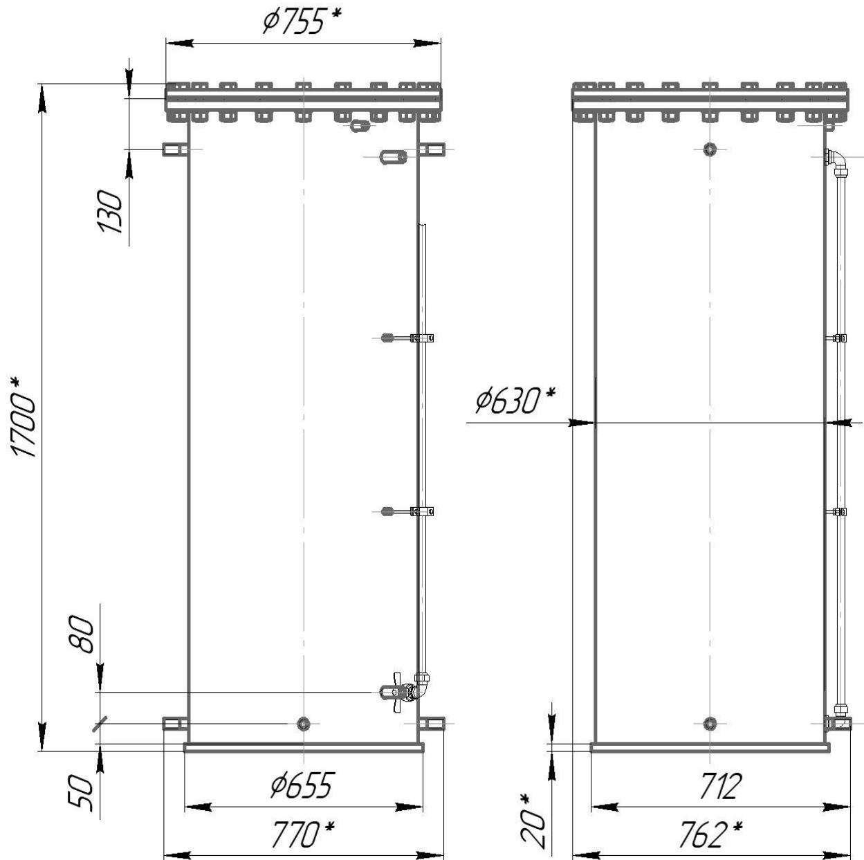
Рис. 1 - Бак для воды БВ-0,45. Общий вид (с УУЖ – дополнительная комплектация).
