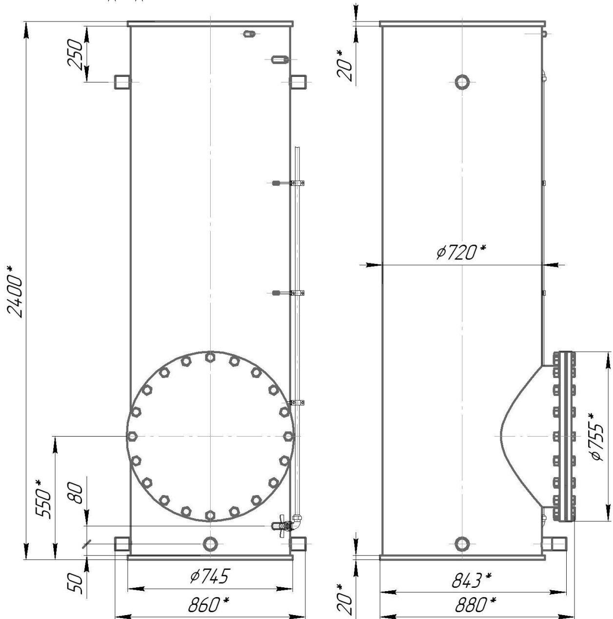
Рис. 1 - Бак для воды БВ-0,9БГ. Общий вид (с УУЖ – дополнительная комплектация).
