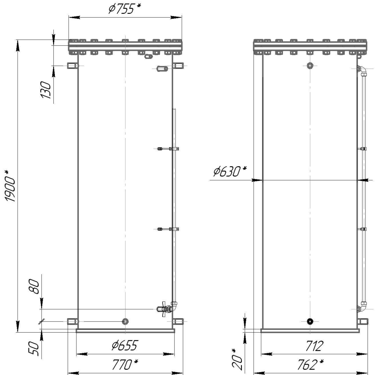
Рис. 1 - Бак для воды БВ-0,5. Общий вид (с УУЖ – дополнительная комплектация).
