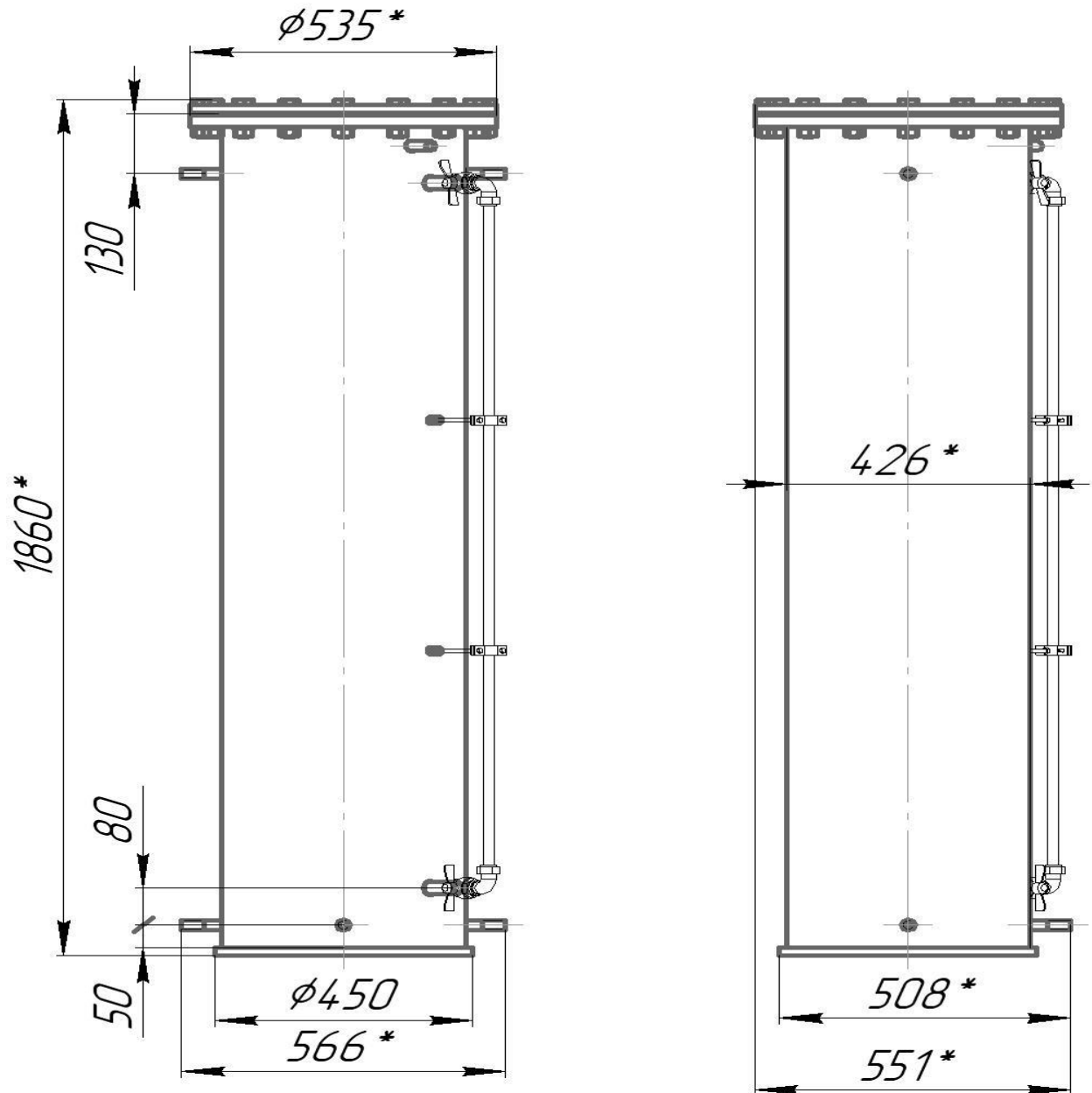
Рис. 1 - Бак для воды БВ-0,25. Общий вид (с УУЖ – дополнительная комплектация).
