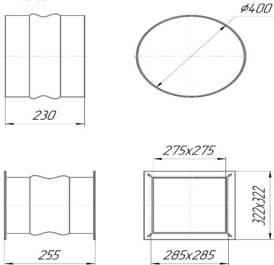
Рис. 1 - Гибкие вставки ГВ-3.
