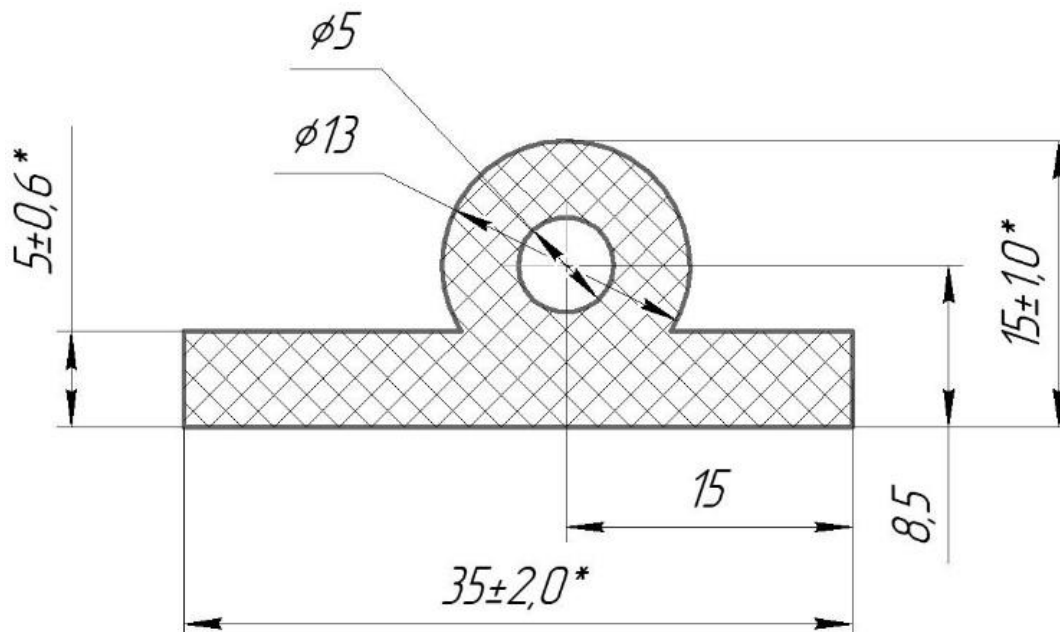
Рис. 1 – Резина уплотнительная (профильная) ТУСМ-4-01. Общий вид
