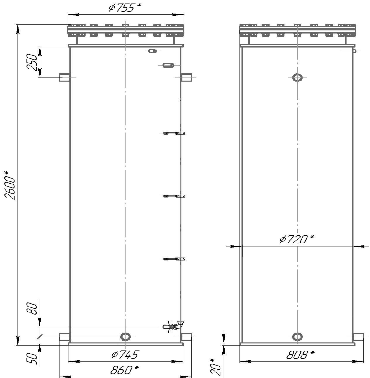
Рис. 1 - Бак для воды БВ-0,9. Общий вид (с УУЖ – дополнительная комплектация).
