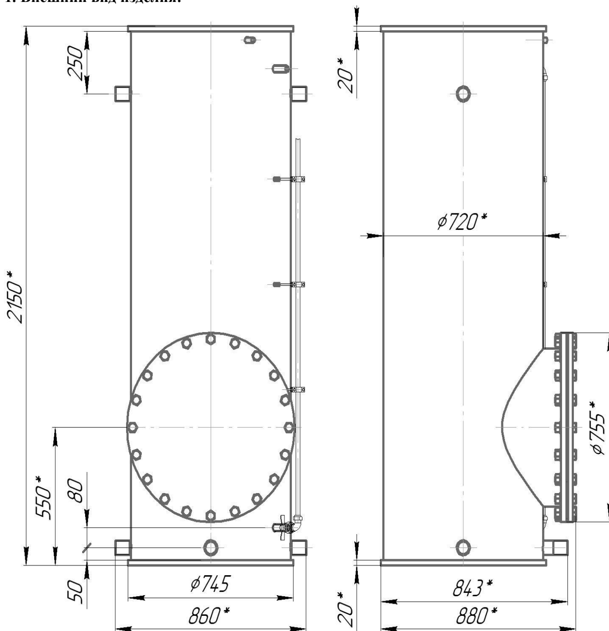
Рис. 1 - Бак для воды БВ-0,8БГ. Общий вид (с УУЖ – дополнительная комплектация).
